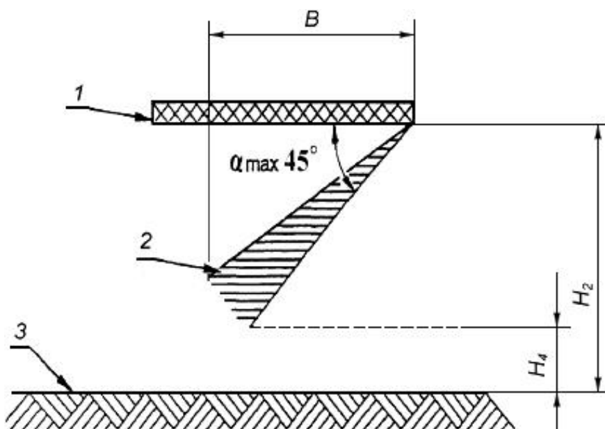
Рисунок 10 - Размеры защитной юбки карусели с расстоянием от нижней плоскости платформы до поверхности игровой площадки H(2) > 400 мм
