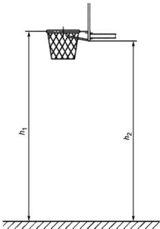
Рисунок 7 - Высота установки корзины для баскетбольного оборудования классов A-D
