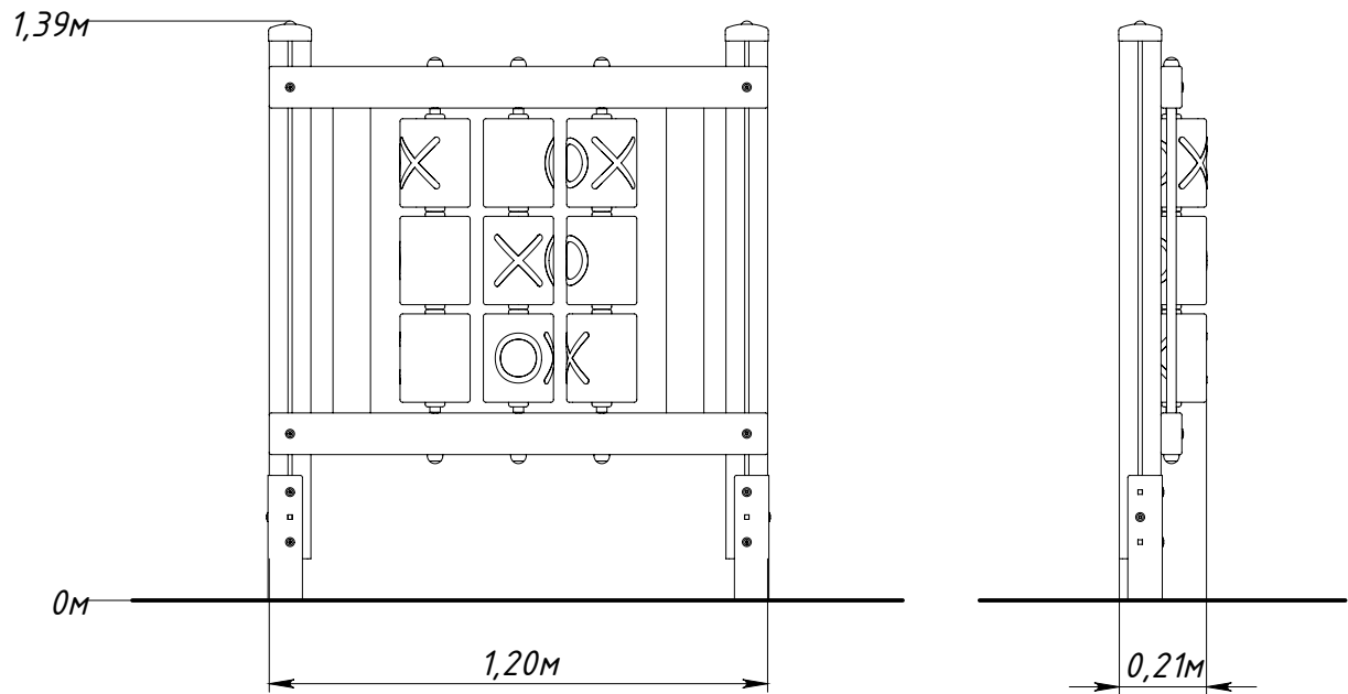
Рисунок 1 — Основные габаритные размеры
