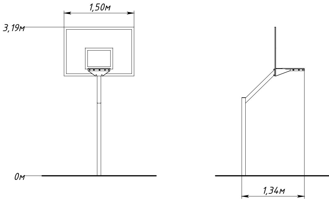
Рисунок 1 — Основные габаритные размеры
