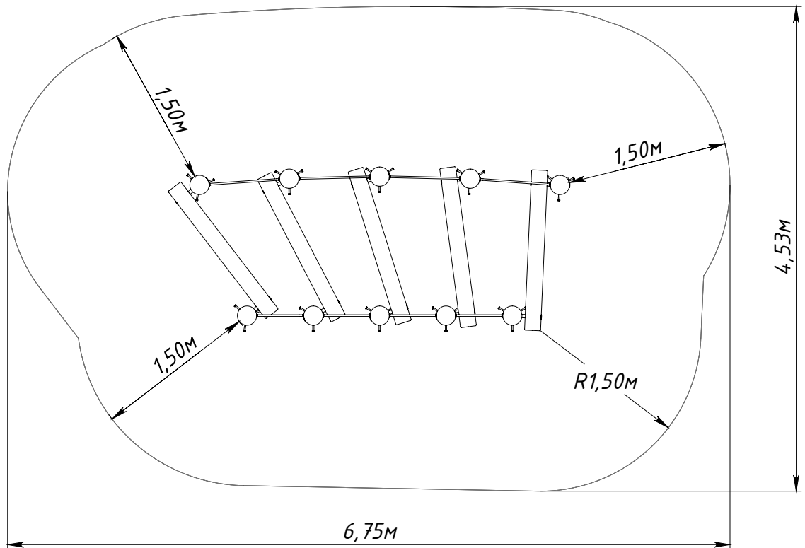
Рисунок 1 — Основные габаритные размеры
